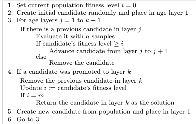
(b) (k + 1) LES Pseudocode
